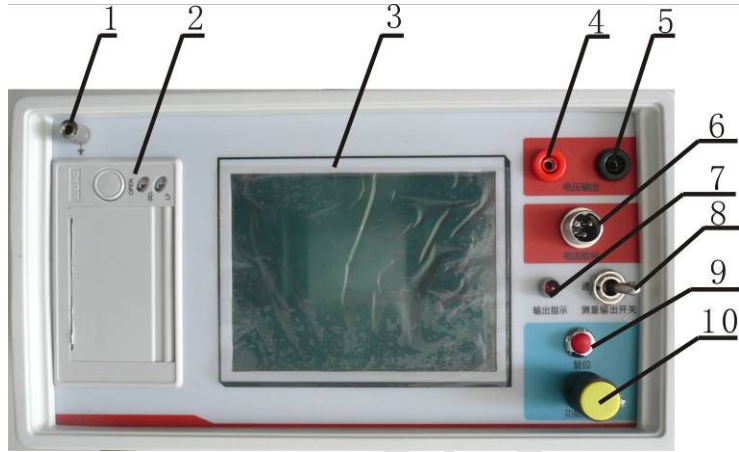
图 2 仪器面板图
