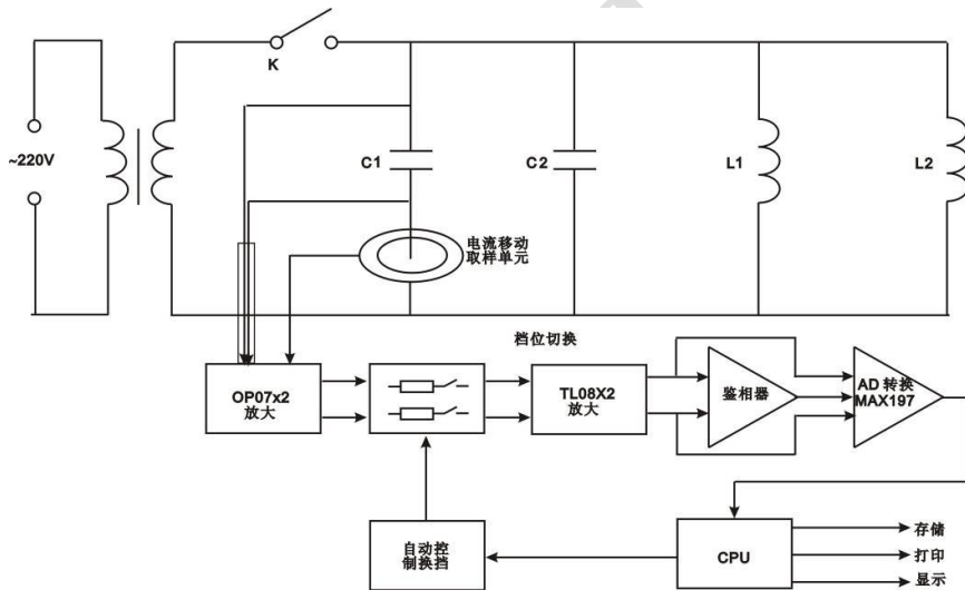
图 1 工作原理图
