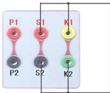
图 3、直阻校零接线图
