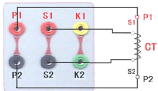
图 4、CT 励磁/直阻/变比/极性/角差/比差试验接线图
