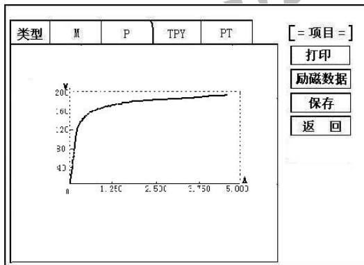
图 22, PT 励磁特性测试结果界面
